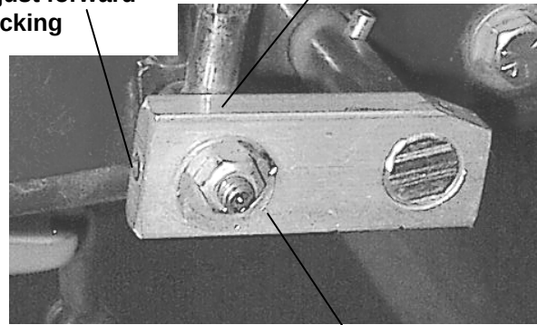
Loosen Nut
