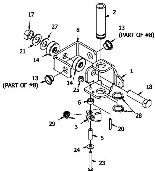
YOKE, SWIVEL ASS'Y (625-169A)
