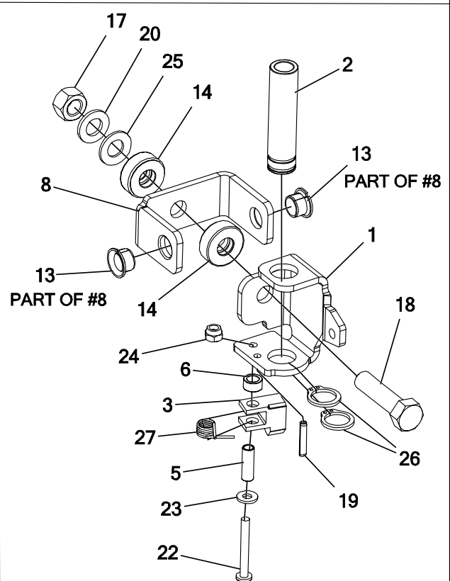
YOKE, SWIVEL, ASS'Y (625-169A)
